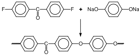
الشكل (3-6): تكاتف 4،4'-ثنائي فلوروثنائي فينيل كيتون مع هيدروكينون
